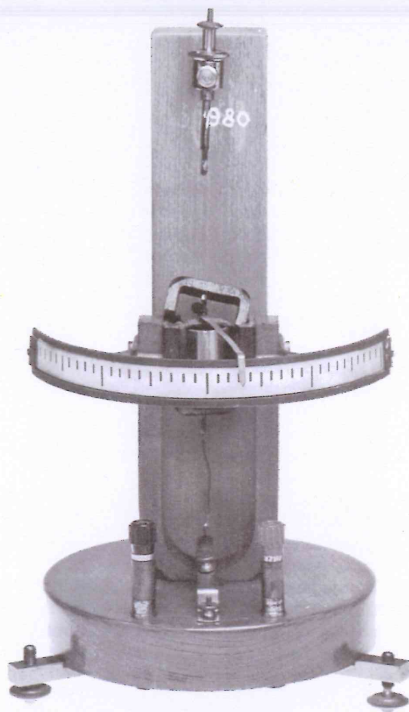
Misuratore elettromagnetico
